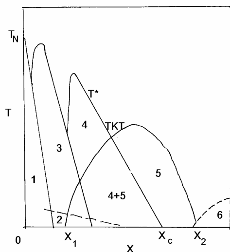
Рис. 4. Фазовая диаграмма температура – кислородный индекс [23]: X_1 , X_c , X_2 – точки квантовых фазовых переходов; ТКТ – тетракритическая точка; 1 – трехмерный антиферромагнетик; 2 – фаза спиновой стеклы; 3 – конкурирующие фазы; 4 – псевдощелевая фаза ( d -волна спиновой плотности); 5 – сверхпроводящая d -фаза; 6 – фаза ферромагнитных корреляций
