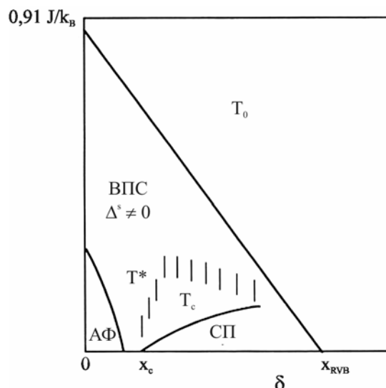
Рис. 3. Фазовая диаграмма системы YBCO [21]:
