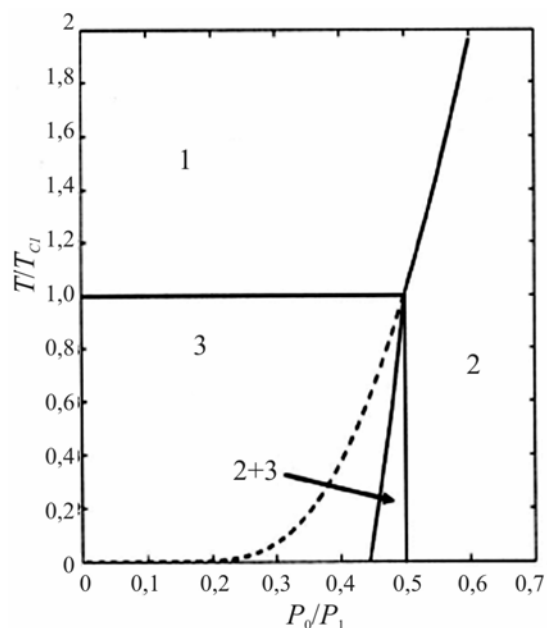
Рис. 1. Расчетная фазовая диаграмма [13]: 1 – область нормального металла; 2 – область ВЗП; 3 – область НВЗП; 2+3 – область расслоения ВЗП + НВЗП; T_{c1} – температура перехода; P_0/P_1 – отношение концентрационных коэффициентов для ВЗП и НВЗП. Пунктирная линия – расчетное положение границы ВЗП – нормальный металл при отсутствии фазы НВЗП
