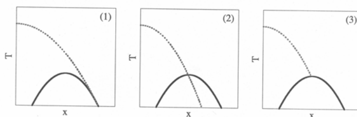
Рис. 1. Различные виды фазовой диаграммы купрата. Сплошные линии – сверхпроводящий «колокол», пунктирные – граница псевдощелевой фазы T^*
