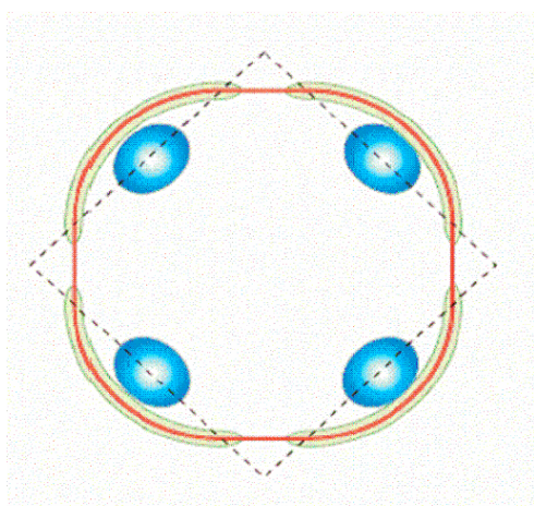
Рис. 3. Поверхность Ферми в передопированных (сплошная линия) и недодопированных (четыре «пятна») купратах (согласно работе [3]). Отдельно показаны фермиевские дуги. Пунктирная линия соединяет точки (k_x, k_y) = (\pm \pi, 0) и (0, \pm \pi) в двумерной зоне Бриллюэна
