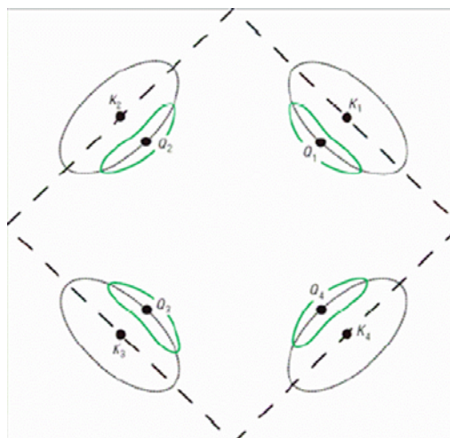
Рис. 4. Электронные карманы ( Q_1 - Q_4 ) на поверхности Ферми [13]
