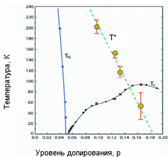
Рис. 2. Граница псевдощелевой фазы ( T^* ) по измерениям эффекта Керра [8]
