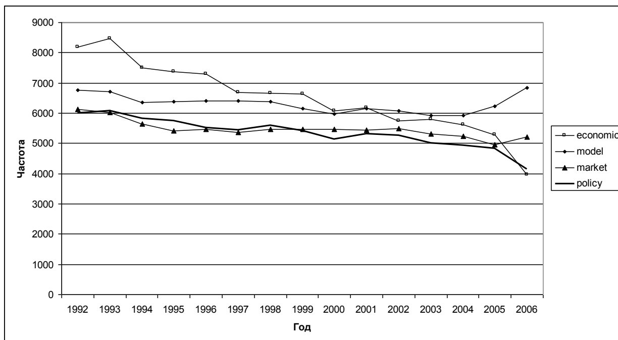
Рис. 6А1. Изменение частот первых четырех терминов по годам (в расчете на 1 млн словоупотреблений)
