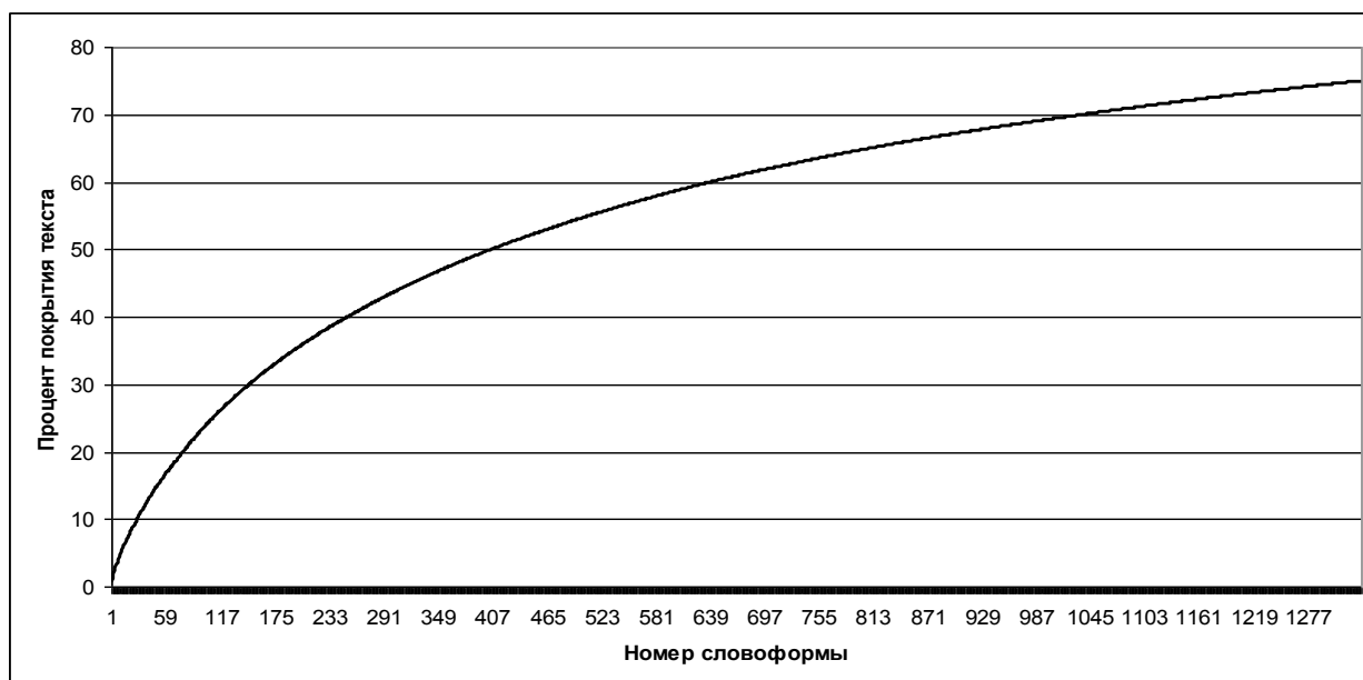
Рис. 6А2. Зависимость степени покрытия текста от числа терминов
